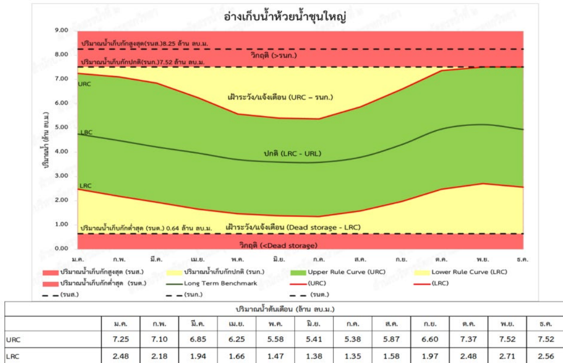
รูปที่ 4.4.2-14 เกณฑ์ปฏิบัติงานอ่างเก็บน้ำแบบพลวัตอ่างเก็บน้ำห้วยน้ำขุนใหญ่
