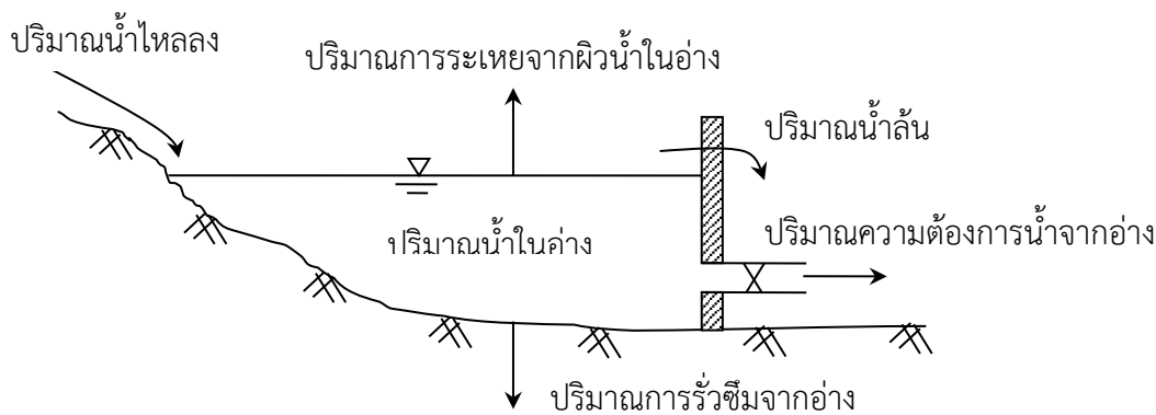
รูปที่ 4.4.2-1 สมดุลของน้ำในอ่างเก็บน้ำ
