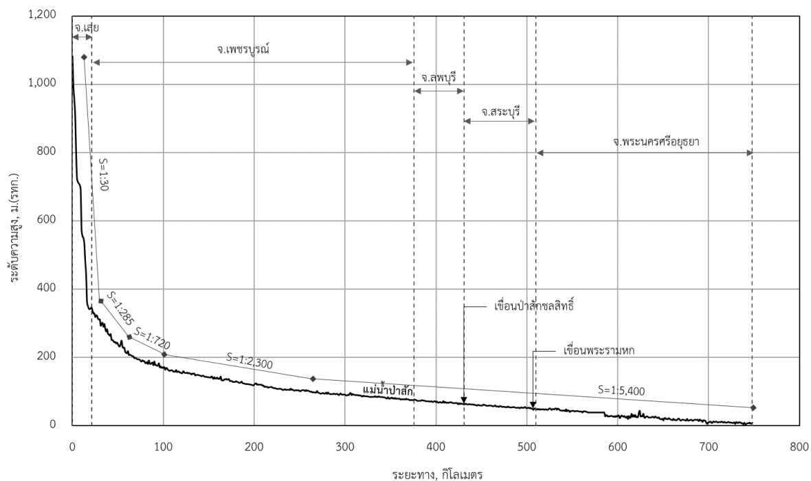
รูปที่ 2.1.1-2 รูปตัดตามยาวแม่น้ำป่าสักแสดงความลาดชันลุ่มน้ำ
