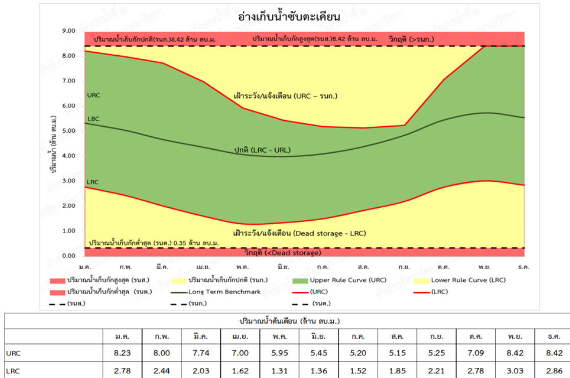
รูปที่ 4.4.2-16 เกณฑ์ปฏิบัติงานอ่างเก็บน้ำแบบพลวัตอ่างเก็บน้ำซับตะเคียน
