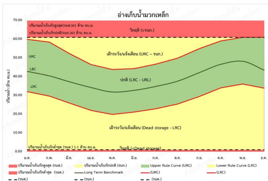
รูปที่ 4.4.2-20 เกณฑ์ปฏิบัติงานอ่างเก็บน้ำแบบพลวัตอ่างเก็บน้ำบ้านดง
