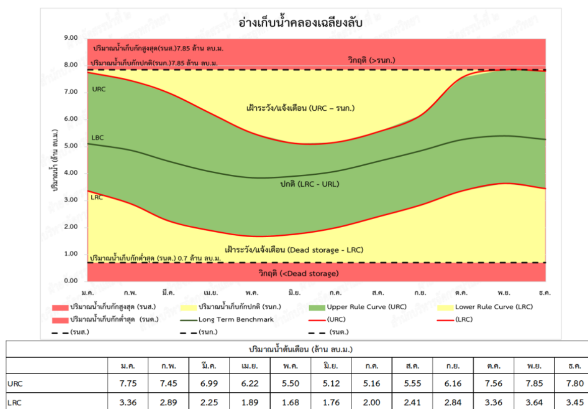
รูปที่ 4.4.2-7 เกณฑ์ปฏิบัติงานอ่างเก็บน้ำแบบพลวัตอ่างเก็บน้ำคลองเจ็ดยักษ์
