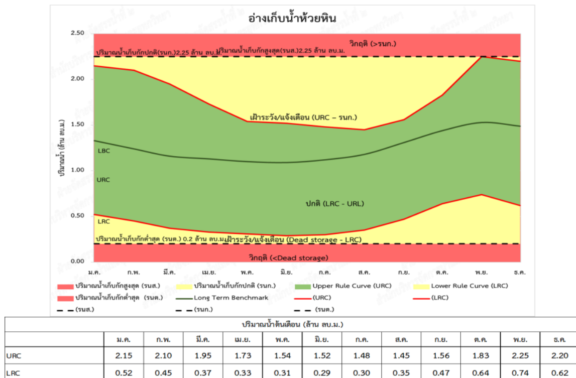
รูปที่ 4.4.2-19 เกณฑ์ปฏิบัติงานอ่างเก็บน้ำแบบพลวัตอ่างเก็บน้ำห้วยหิน
