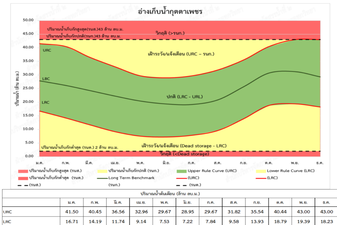
รูปที่ 4.4.2-17 เกณฑ์ปฏิบัติงานอ่างเก็บน้ำแบบพลวัตอ่างเก็บน้ำกุดตาเพชร
