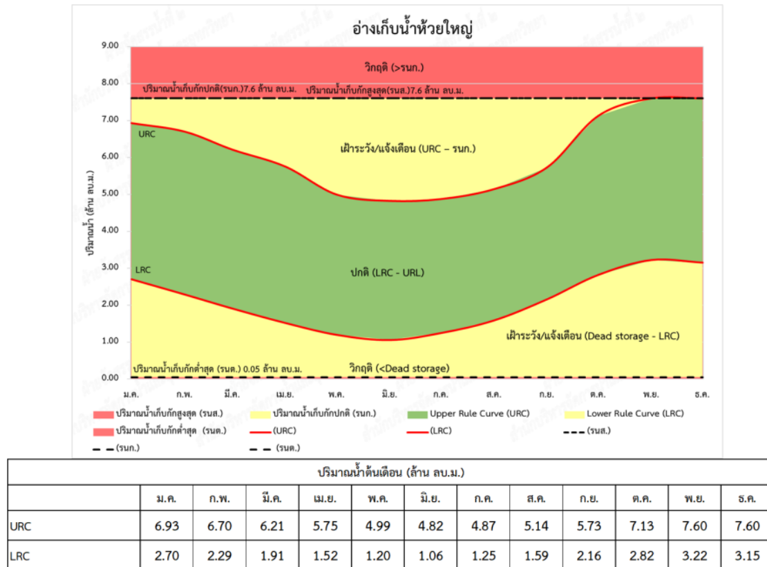
รูปที่ 4.4.2-18 เกณฑ์ปฏิบัติงานอ่างเก็บน้ำแบบพลวัตอ่างเก็บน้ำห้วยใหญ่
