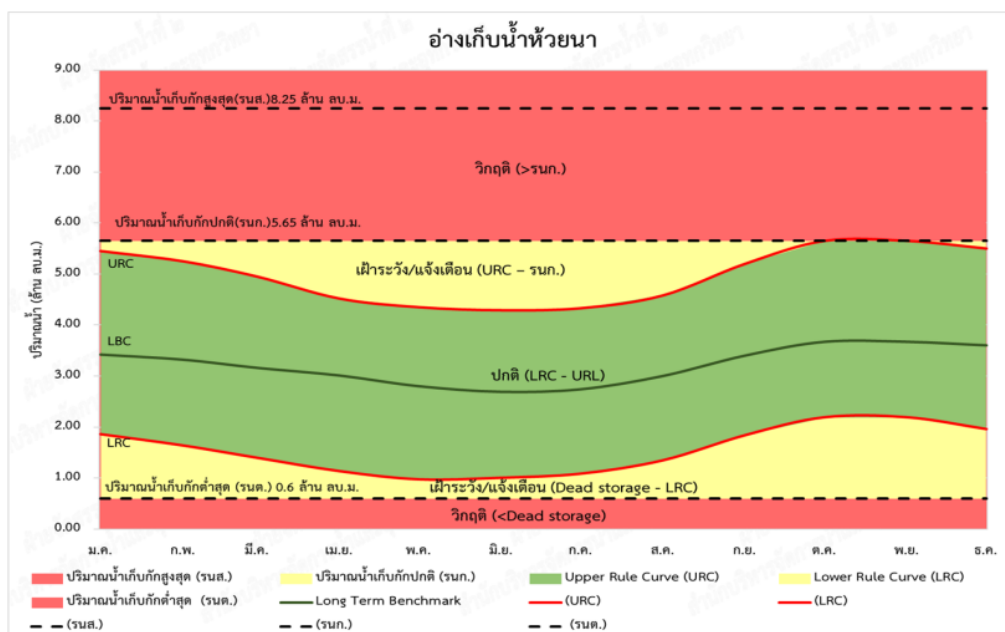
รูปที่ 4.4.2-8 เกณฑ์ปฏิบัติงานอ่างเก็บน้ำแบบพลวัตอ่างเก็บน้ำคลองเพรียว
