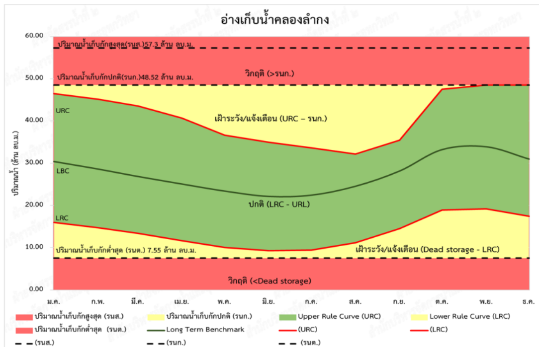
รูปที่ 4.4.2-12 เกณฑ์ปฏิบัติงานอ่างเก็บน้ำแบบพลวัตอ่างเก็บน้ำห้วยน้ำก่อ
