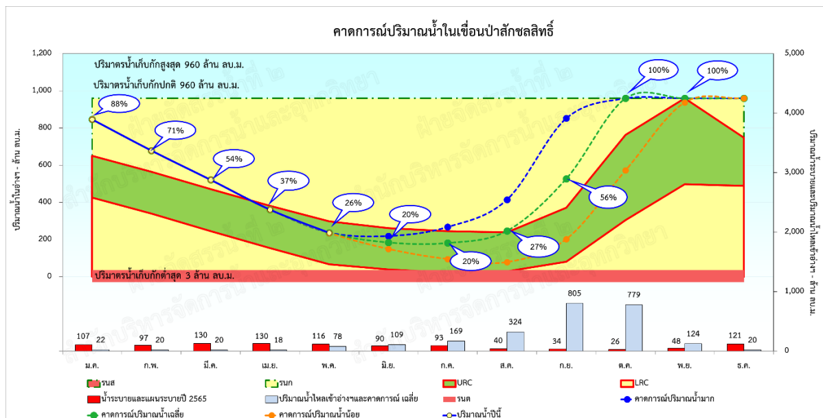
รูปที่ 4.4.2-6 การปฏิบัติงานอ่างเก็บน้ำเขื่อนป่าสักชลสิทธิ์ร่วมกับการคาดการณ์ปริมาณน้ำ พ.ศ.2566
