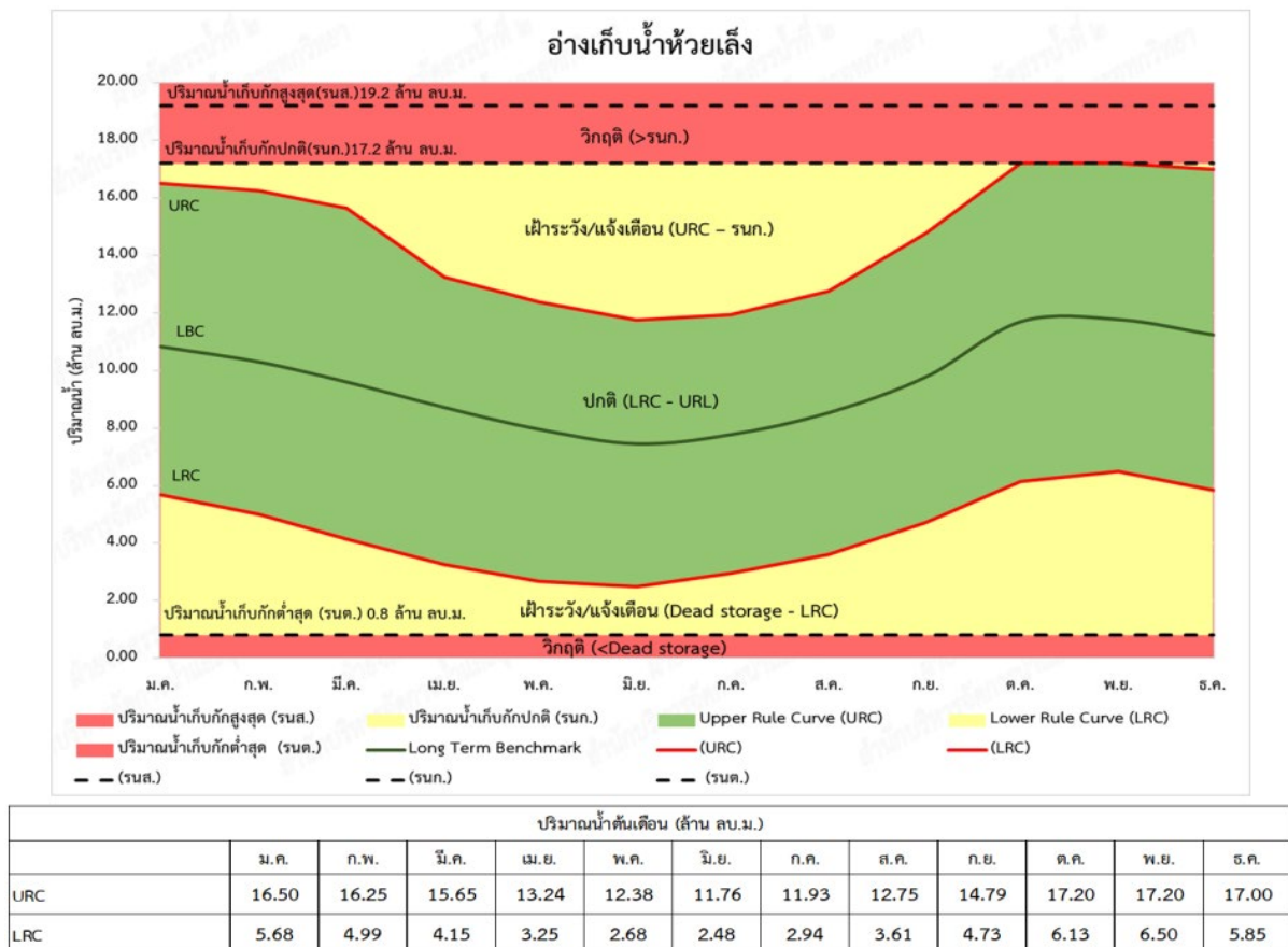
รูปที่ 4.4.2-15 เกณฑ์ปฏิบัติงานอ่างเก็บน้ำแบบพลวัตอ่างเก็บน้ำห้วยเล้ง
