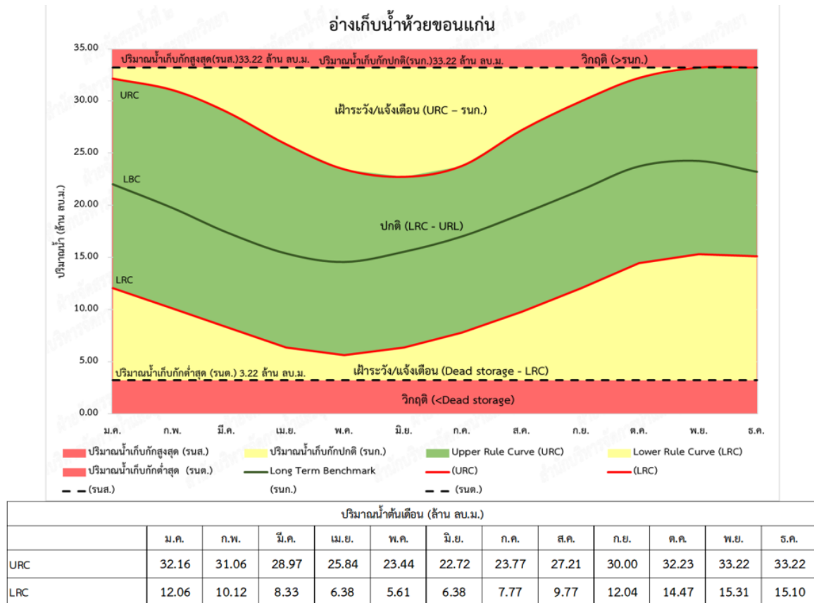
รูปที่ 4.4.2-10 เกณฑ์ปฏิบัติงานอ่างเก็บน้ำแบบพลวัตอ่างเก็บน้ำห้วยขอนแก่น
