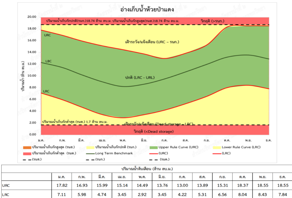
รูปที่ 4.4.2-11 เกณฑ์ปฏิบัติงานอ่างเก็บน้ำแบบพลวัตอ่างเก็บน้ำห้วยป่าแดง
