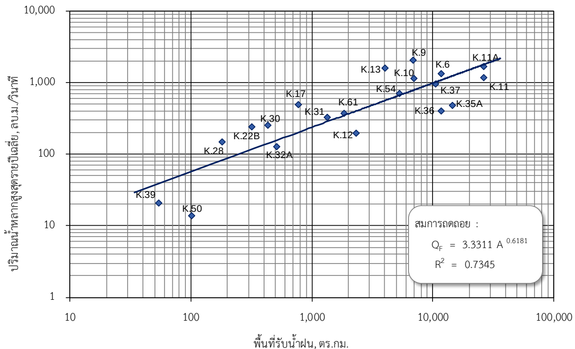
รูปที่ 2.1.4-6 กราฟแสดงความสัมพันธ์ระหว่างปริมาณน้ำหลากสูงสุดรายปีเฉลี่ยและพื้นที่รับน้ำฝน
