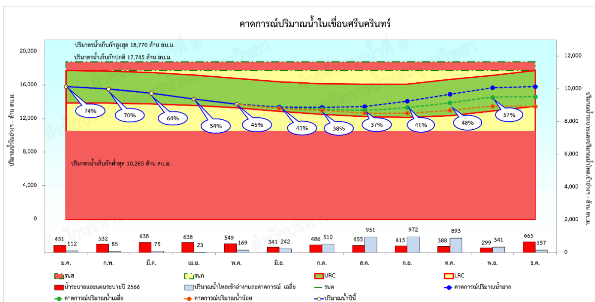
รูปที่ 4.4.2-6 เกณฑ์ปฏิบัติงานอ่างเก็บน้ำแบบพลวัตอ่างเก็บน้ำศรีนครินทร์
