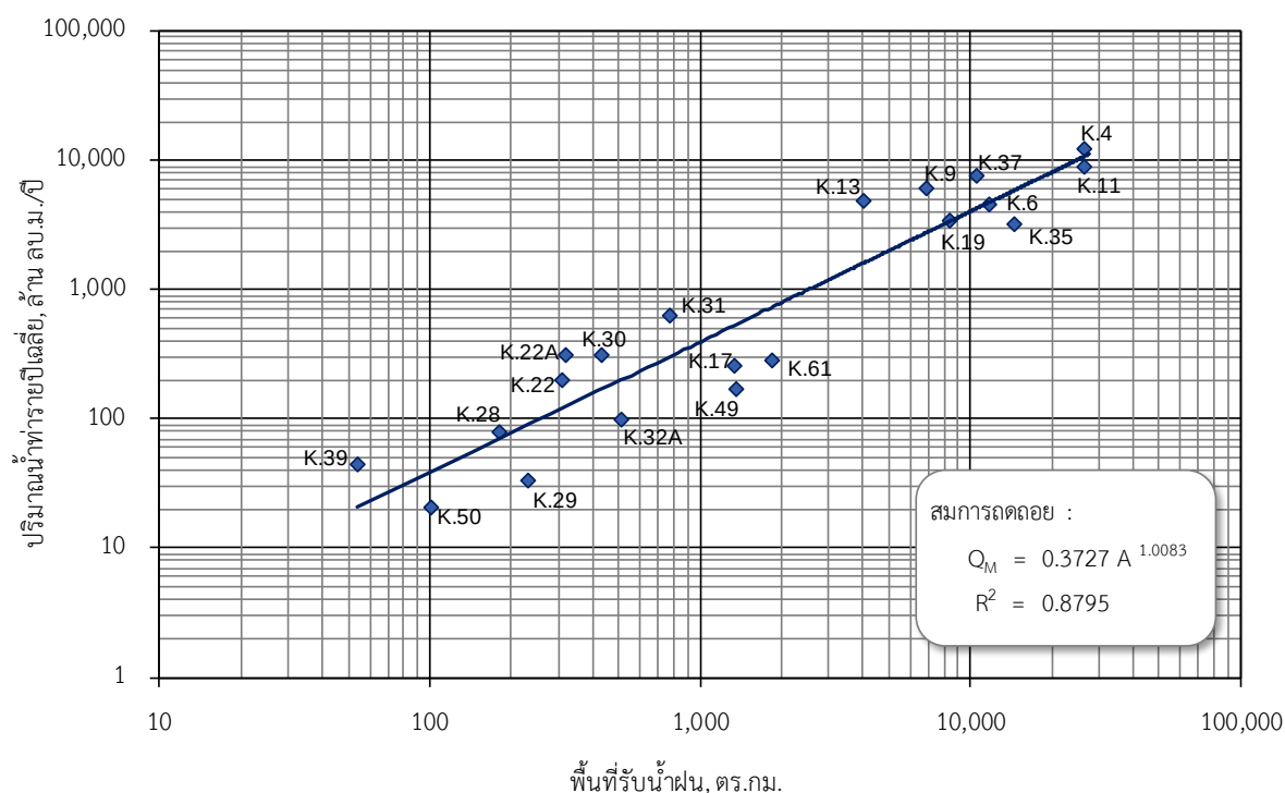
รูปที่ 2.1.4-5 กราฟแสดงความสัมพันธ์ระหว่างปริมาณน้ำท่ารายปีเฉลี่ยและพื้นที่รับน้ำฝน
