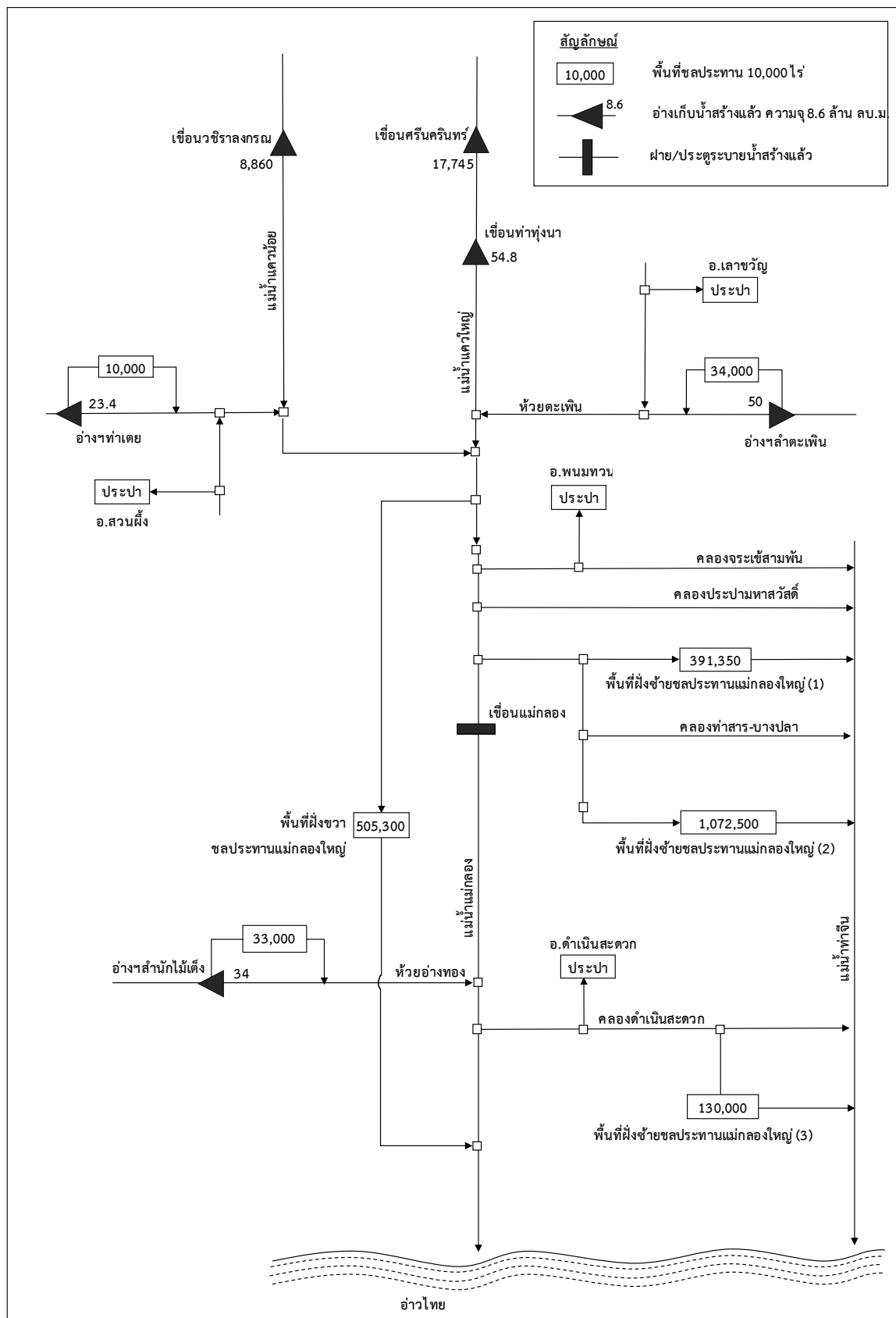
รูปที่ 2.1.3-2 แผนผังระบบลุ่มน้ำแม่กลอง
