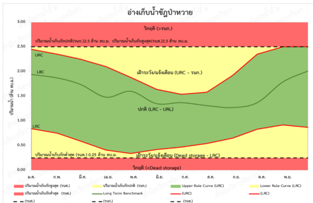
รูปที่ 4.4.2-9 เกณฑ์ปฏิบัติงานอ่างเก็บน้ำแบบพลวัตอ่างเก็บน้ำห้วยพุเตย
