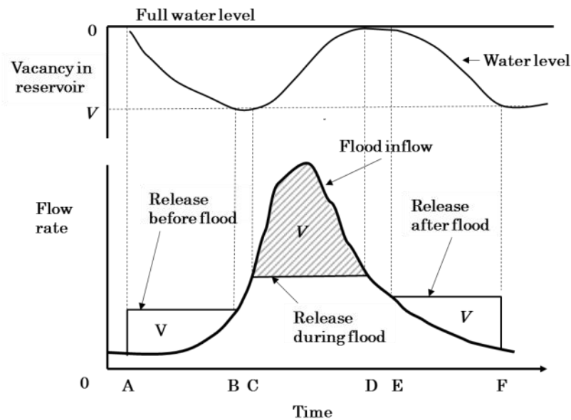
รูปที่ 4.4.2-3 กระบวนการของระบบปฏิบัติการอ่างเก็บน้ำ
