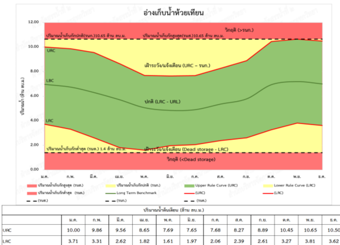
รูปที่ 4.4.2-8 เกณฑ์ปฏิบัติงานอ่างเก็บน้ำแบบพลวัตอ่างเก็บน้ำห้วยเทียน
