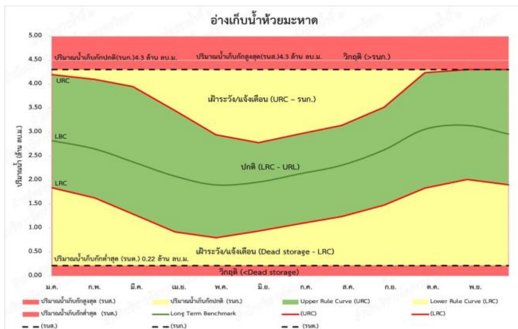
รูปที่ 4.4.2-11 เกณฑ์ปฏิบัติงานอ่างเก็บน้ำแบบพลวัตอ่างเก็บน้ำห้วยสำนักไม้เต็ง
