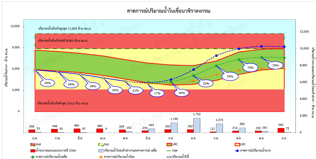
รูปที่ 4.4.2-5 เกณฑ์ปฏิบัติงานอ่างเก็บน้ำแบบพลวัตอ่างเก็บน้ำวชิราลงกรณ์
