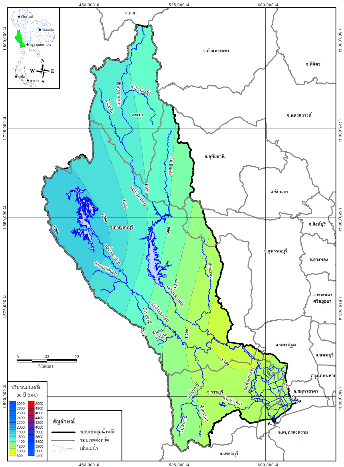
รูปที่ 2.1.4-3 เส้นชั้นน้ำฝนรายปีเฉลี่ยลุ่มน้ำแม่กลอง
