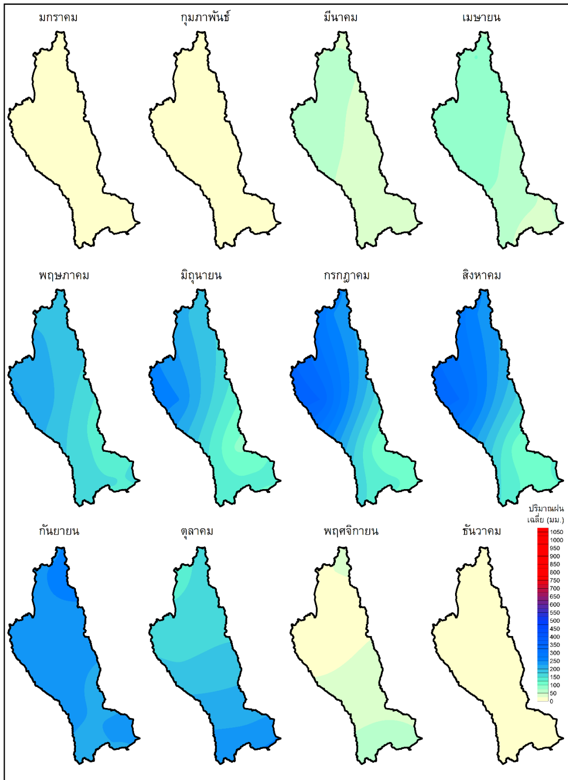
รูปที่ 2.1.4-4 เส้นชั้นน้ำฝนรายเดือนเฉลี่ยลุ่มน้ำแม่กลอง
