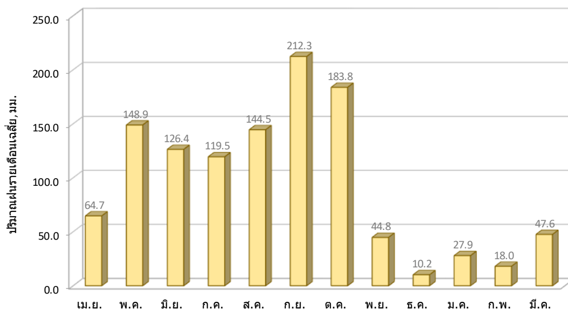
รูปที่ 2.1.4-1 การกระจายปริมาณฝนรายเดือนเฉลี่ยลุ่มน้ำแม่กลอง
