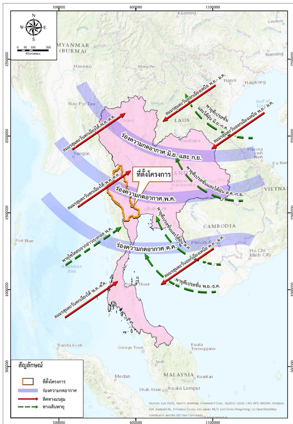
รูปที่ 2.1.2-1 ทิศทางและช่วงเวลาการเกิดของลมมรสุมและลมพายุที่พัดเข้าสู่ประเทศไทย
