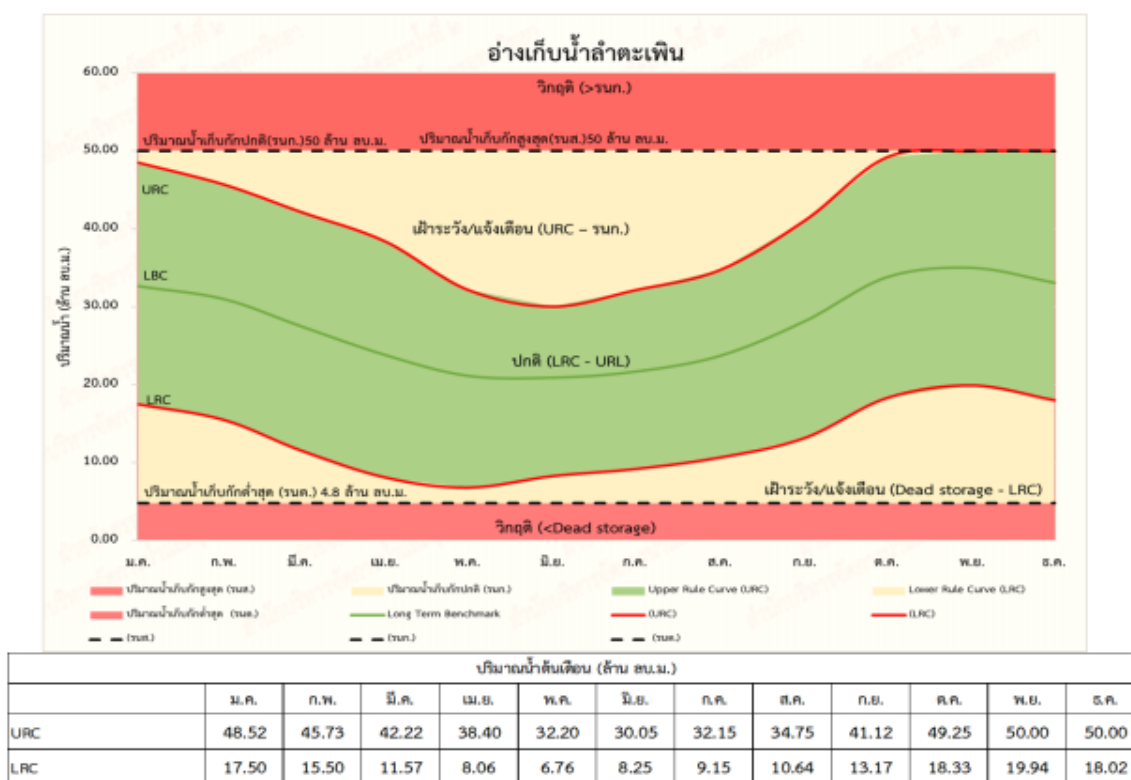
รูปที่ 4.4.2-7 เกณฑ์ปฏิบัติงานอ่างเก็บน้ำแบบพลวัตอ่างเก็บน้ำลำตะเพิน
