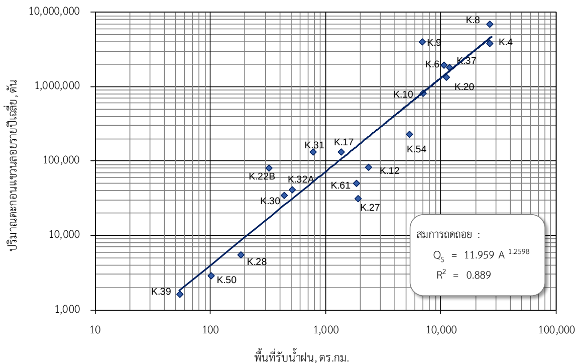
รูปที่ 2.1.4-7 กราฟแสดงความสัมพันธ์ระหว่างปริมาณตะกอนแขวนลอยรายปีเฉลี่ยและพื้นที่รับน้ำฝน
