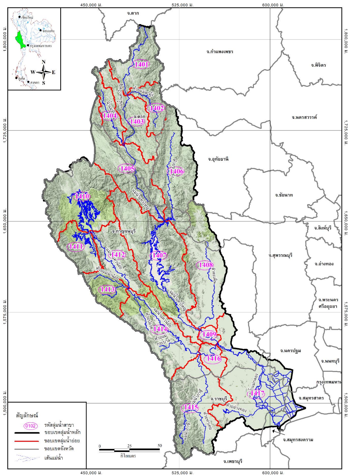
รูปที่ 2.1.3-1 ขอบเขตลุ่มน้ำสาขาในลุ่มน้ำแม่กลอง
