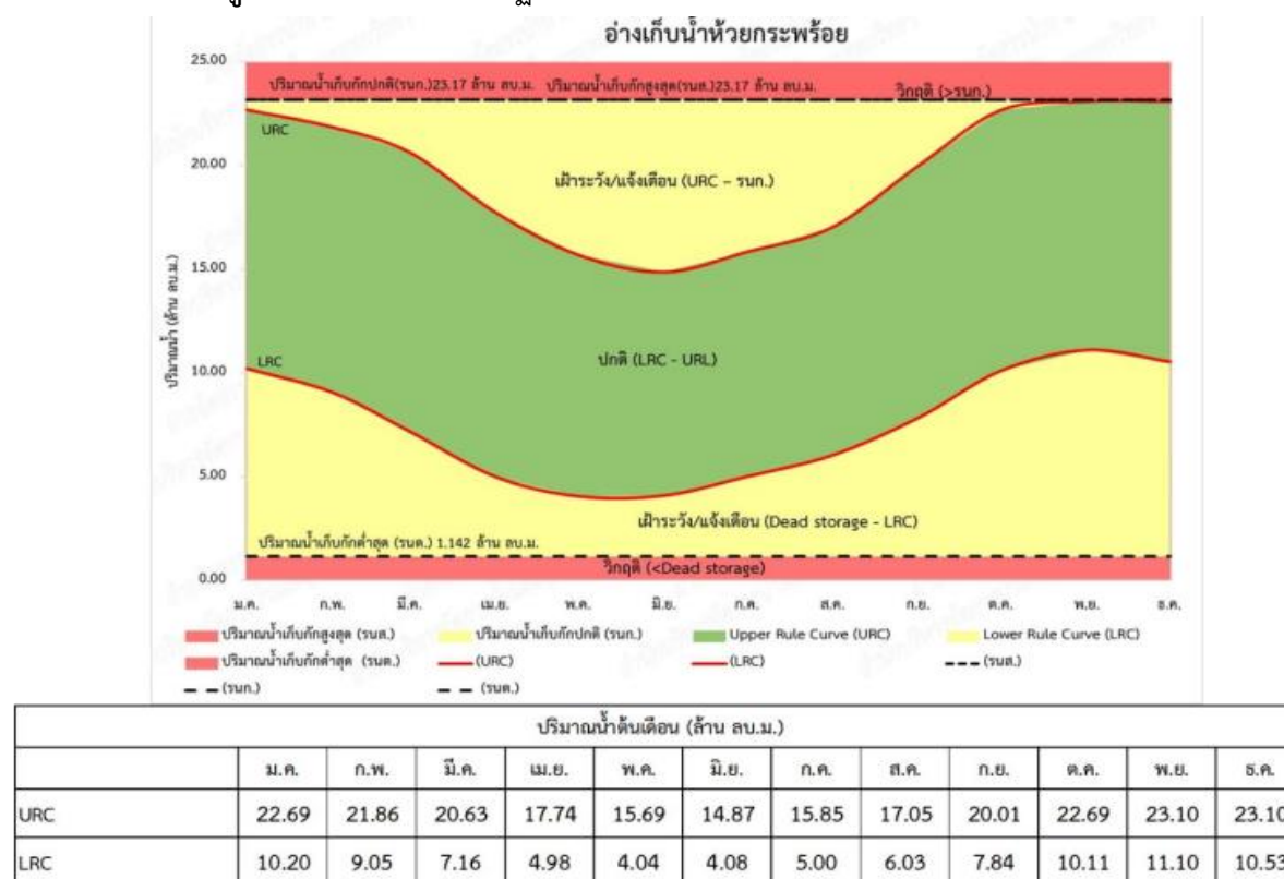
รูปที่ 4.4.2-14 เกณฑ์ปฏิบัติงานอ่างเก็บน้ำแบบพลวัตอ่างเก็บน้ำห้วยกระพ้อ
