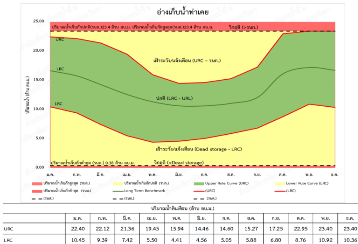
รูปที่ 4.4.2-13 เกณฑ์ปฏิบัติงานอ่างเก็บน้ำแบบพลวัตอ่างเก็บน้ำท่าเคย
