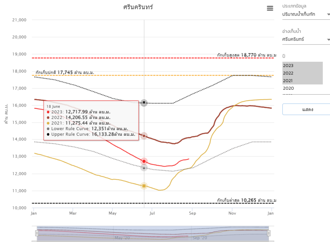
รูปที่ 4.2.2-11 การแสดงข้อมูลปริมาณน้ำในอ่างเก็บน้ำร่วมกับข้อมูลโค้งปฏิบัติงานอ่างเก็บน้ำ
