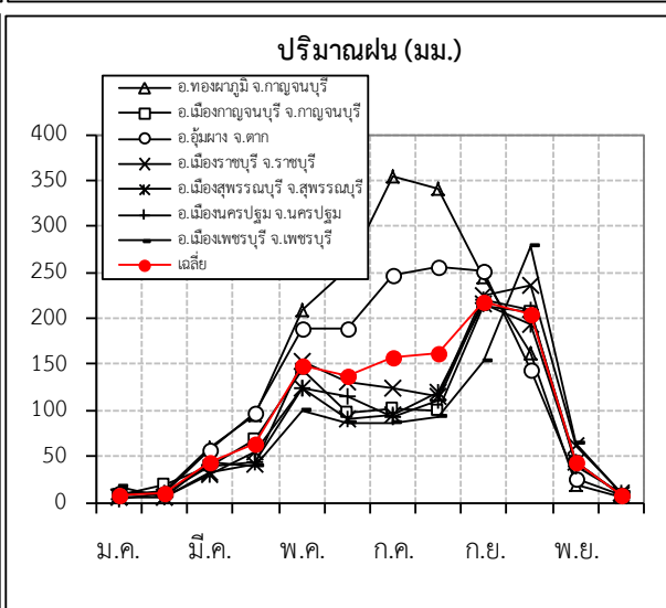
รูปที่ 2.1.2-2 การผันแปรรายเดือนของตัวแปรภูมิอากาศหลักสถานีตรวจอากาศในลุ่มน้ำแม่กลอง
