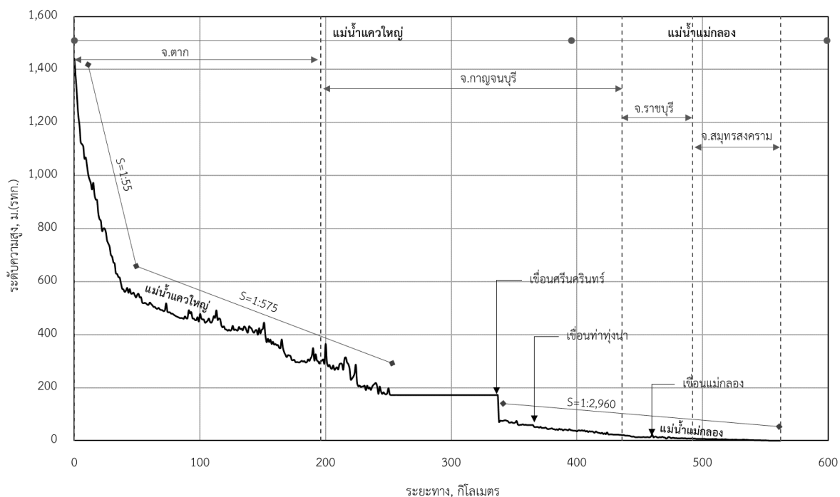
รูปที่ 2.1.1-2 รูปตัดตามยาวแม่น้ำแควใหญ่-แม่กลองแสดงความลาดชันลุ่มน้ำแม่กลอง
