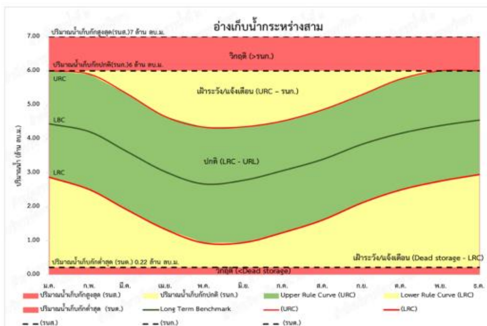
รูปที่ 4.4.2-11 เกณฑ์ปฏิบัติงานอ่างเก็บน้ำแบบพลวัตอ่างเก็บน้ำห้วยตะแปด
