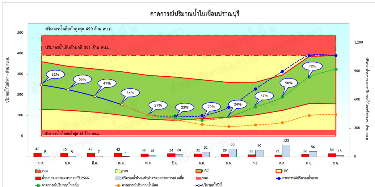
รูปที่ 4.4.2-6 เกณฑ์ปฏิบัติงานอ่างเก็บน้ำแบบพลวัตอ่างเก็บน้ำปราณบุรี
