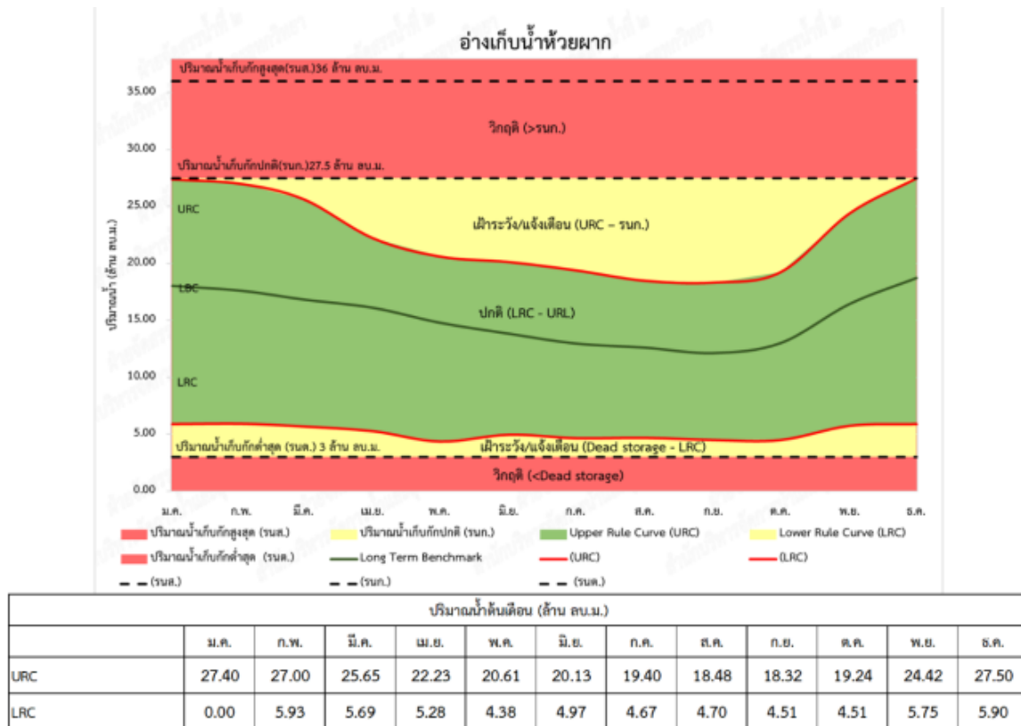
รูปที่ 4.4.2-14 เกณฑ์ปฏิบัติงานอ่างเก็บน้ำแบบพลวัตอ่างเก็บน้ำห้วยผาก
