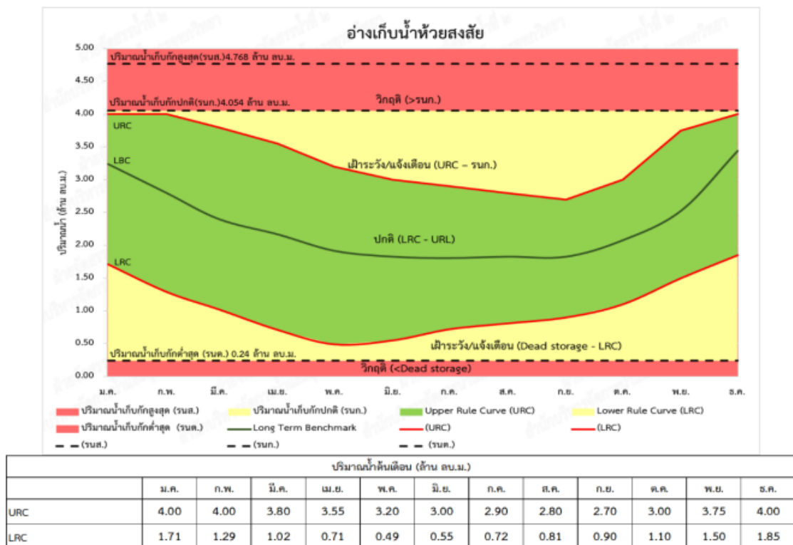
รูปที่ 4.4.2-8 เกณฑ์ปฏิบัติงานอ่างเก็บน้ำแบบพลวัตอ่างเก็บน้ำห้วยสงสัย
