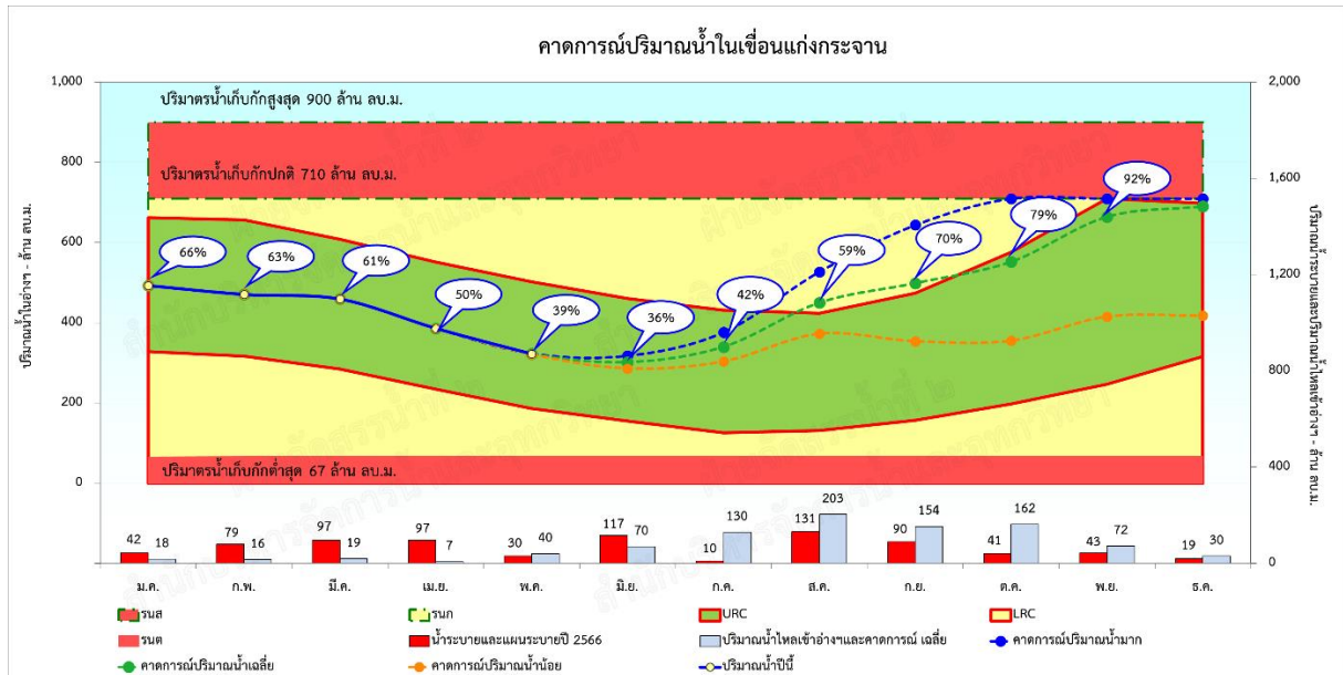
รูปที่ 4.4.2-5 เกณฑ์ปฏิบัติงานอ่างเก็บน้ำแบบพลวัตอ่างเก็บน้ำแก่งกระจาน
