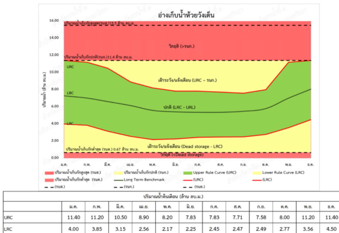
รูปที่ 4.4.2-21 เกณฑ์ปฏิบัติงานอ่างเก็บน้ำแบบพลวัตอ่างเก็บน้ำห้วยวังเต็น
