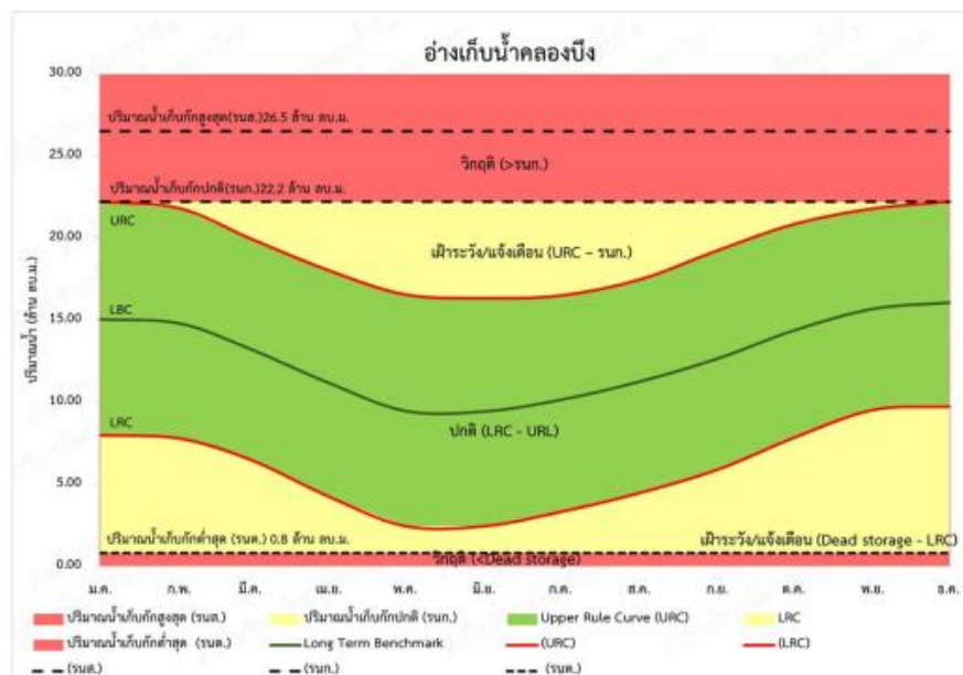
รูปที่ 4.4.2-17 เกณฑ์ปฏิบัติงานอ่างเก็บน้ำแบบพลวัตอ่างเก็บน้ำยางชุม
