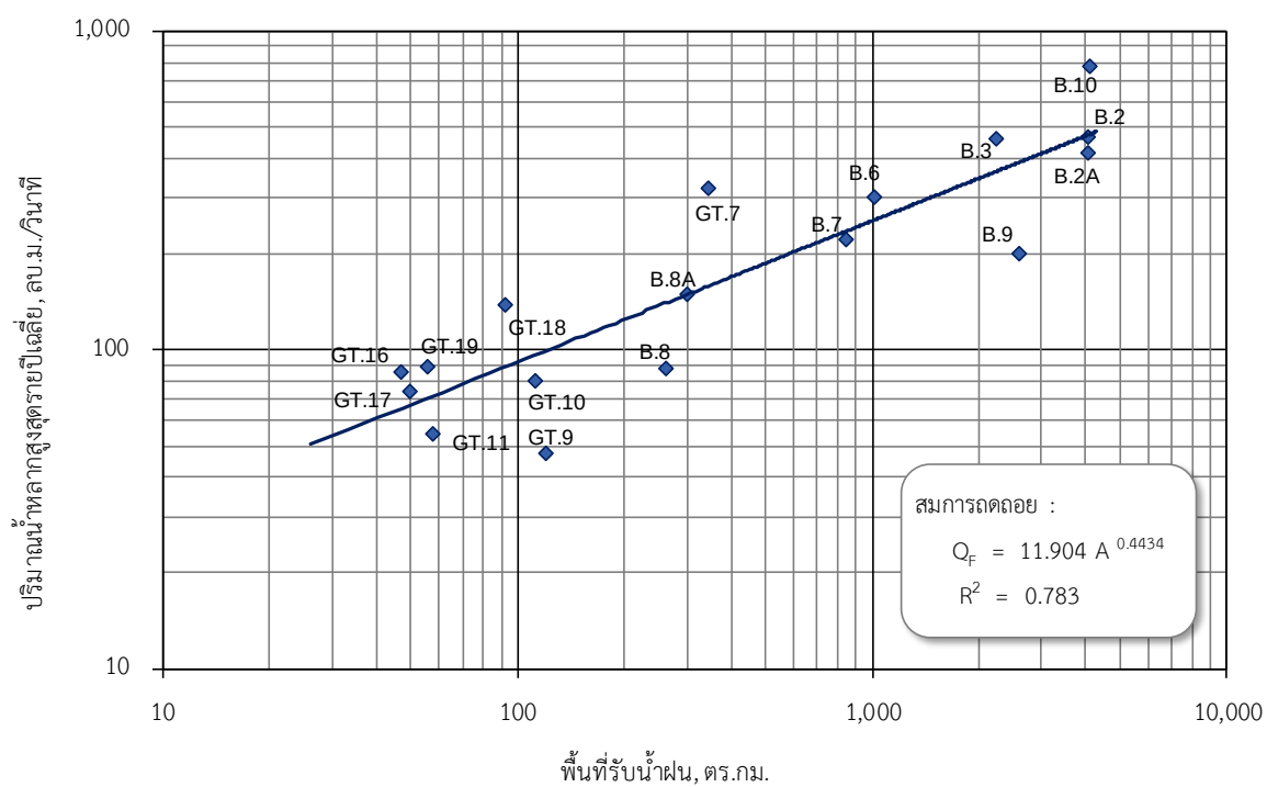
รูปที่ 2.1.4-8 กราฟแสดงความสัมพันธ์ระหว่างปริมาณน้ำหลากสูงสุดรายปีเฉลี่ยและพื้นที่รับน้ำฝน
