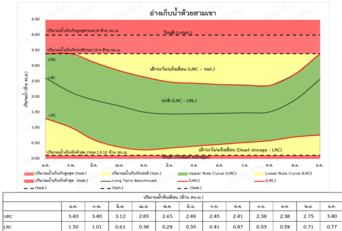
รูปที่ 4.4.2-7 เกณฑ์ปฏิบัติงานอ่างเก็บน้ำแบบพลวัตอ่างเก็บน้ำห้วยสามเขา
