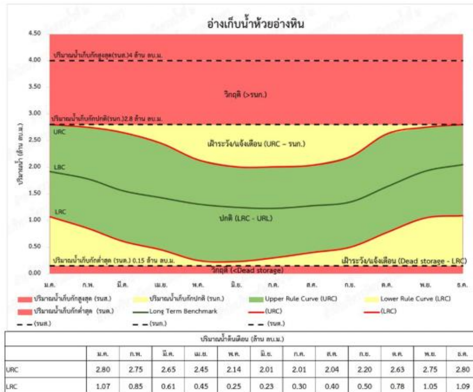
รูปที่ 4.4.2-19 เกณฑ์ปฏิบัติงานอ่างเก็บน้ำแบบพลวัตอ่างเก็บน้ำห้วยอ่างหิน
