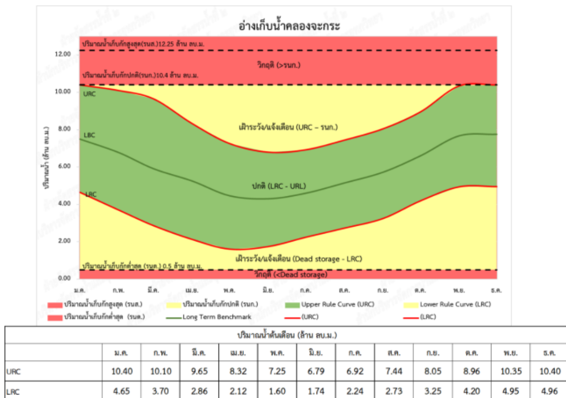
รูปที่ 4.4.2-16 เกณฑ์ปฏิบัติงานอ่างเก็บน้ำแบบพลวัตอ่างเก็บน้ำคลองจะกระ
