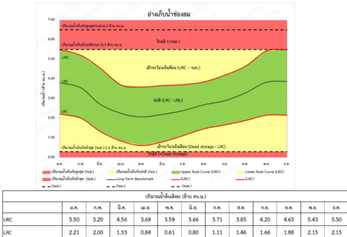
รูปที่ 4.4.2-15 เกณฑ์ปฏิบัติงานอ่างเก็บน้ำแบบพลวัตอ่างเก็บน้ำคลองช่องลม
