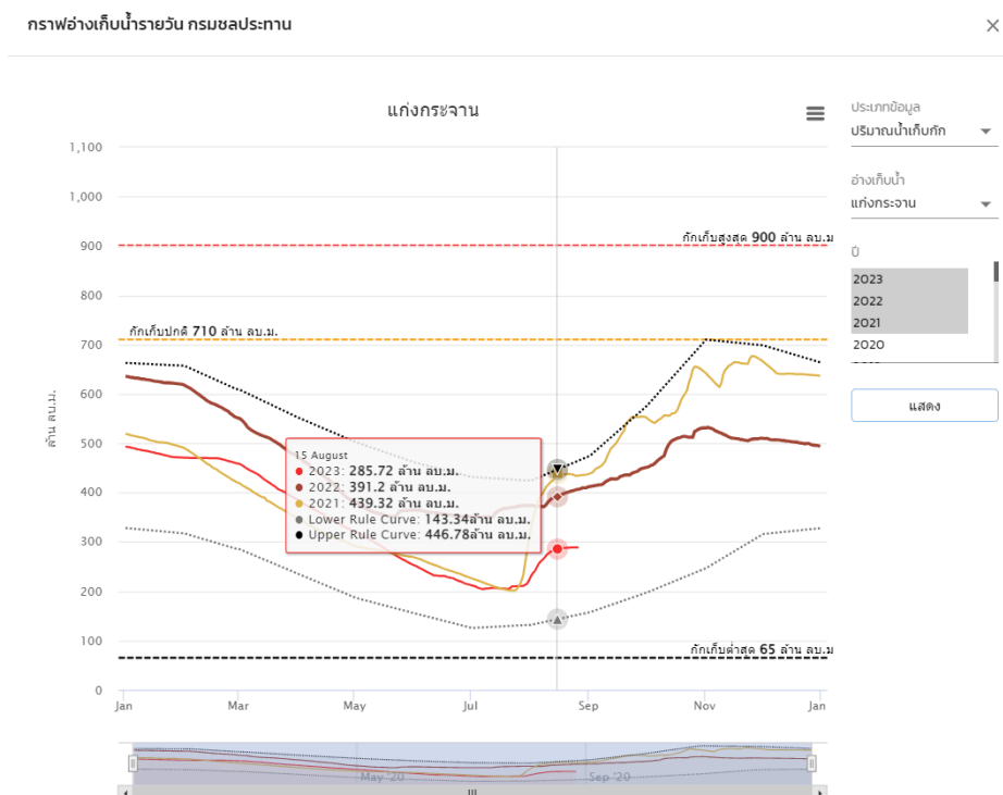
รูปที่ 4.2.2-10 การแสดงข้อมูลปริมาณน้ำในอ่างเก็บน้ำร่วมกับข้อมูลโค้งปฏิบัติงานอ่างเก็บน้ำ
