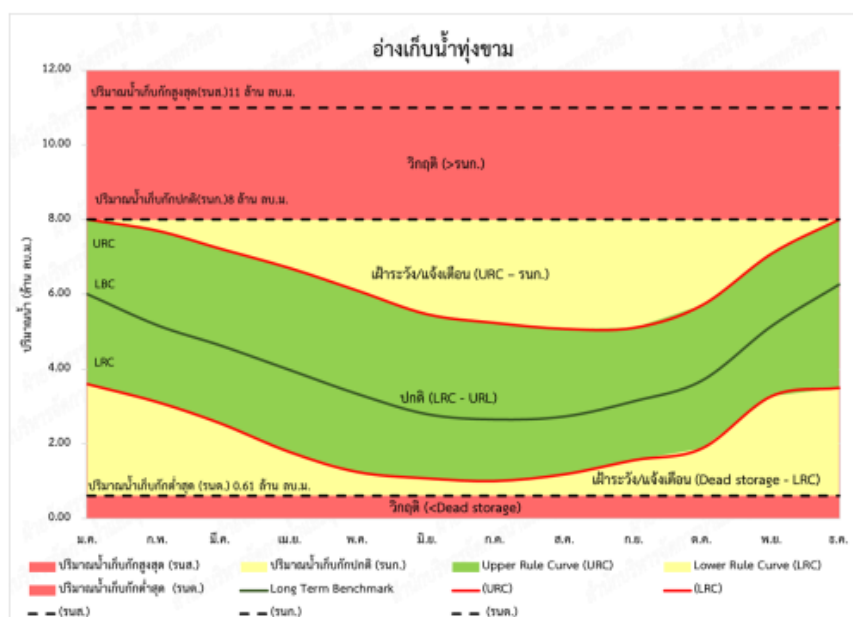
รูปที่ 4.4.2-9 เกณฑ์ปฏิบัติงานอ่างเก็บน้ำแบบพลวัตอ่างเก็บน้ำห้วยทราย
