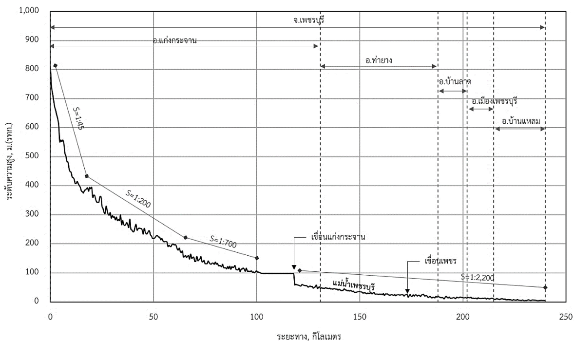
รูปที่ 2.1.1-2 รูปตัดตามยาวแม่น้ำเพชรบุรีแสดงความลาดชันลุ่มน้ำ
