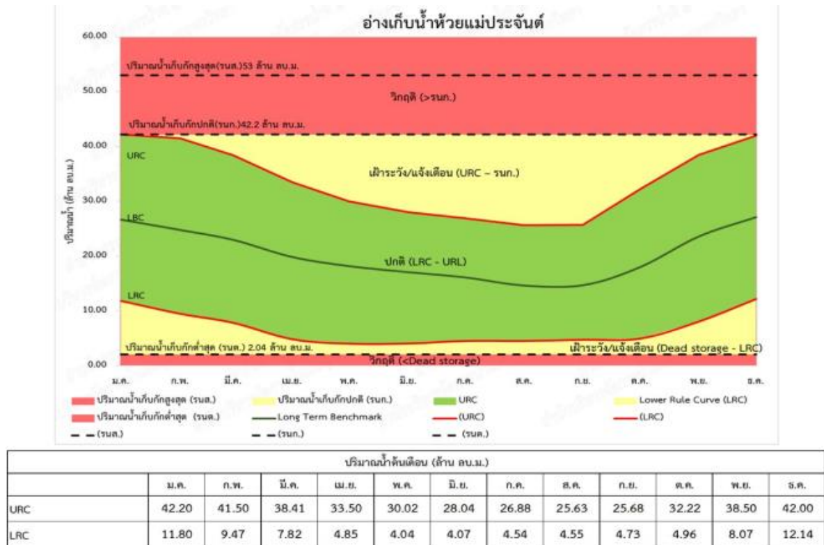
รูปที่ 4.4.2-13 เกณฑ์ปฏิบัติงานอ่างเก็บน้ำแบบพลวัตอ่างเก็บน้ำห้วยแม่ประจันต์
