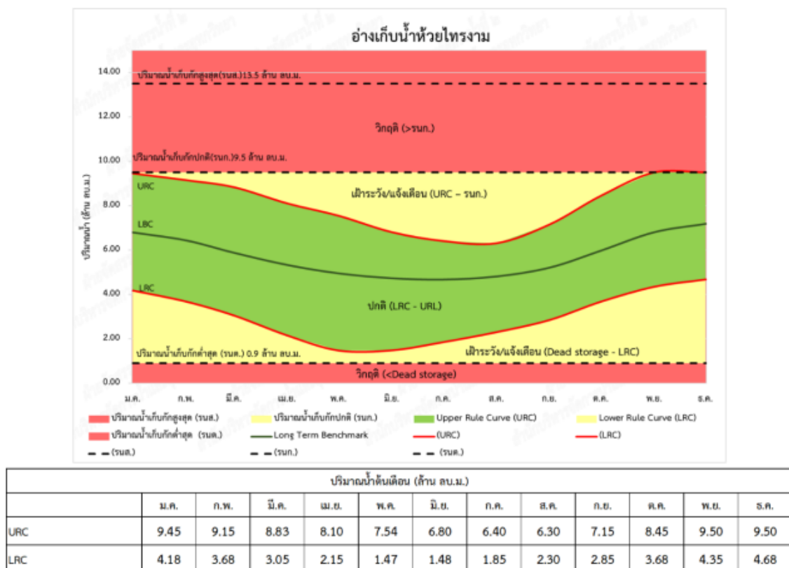
รูปที่ 4.4.2-20 เกณฑ์ปฏิบัติงานอ่างเก็บน้ำแบบพลวัตอ่างเก็บน้ำห้วยไทรงาม
